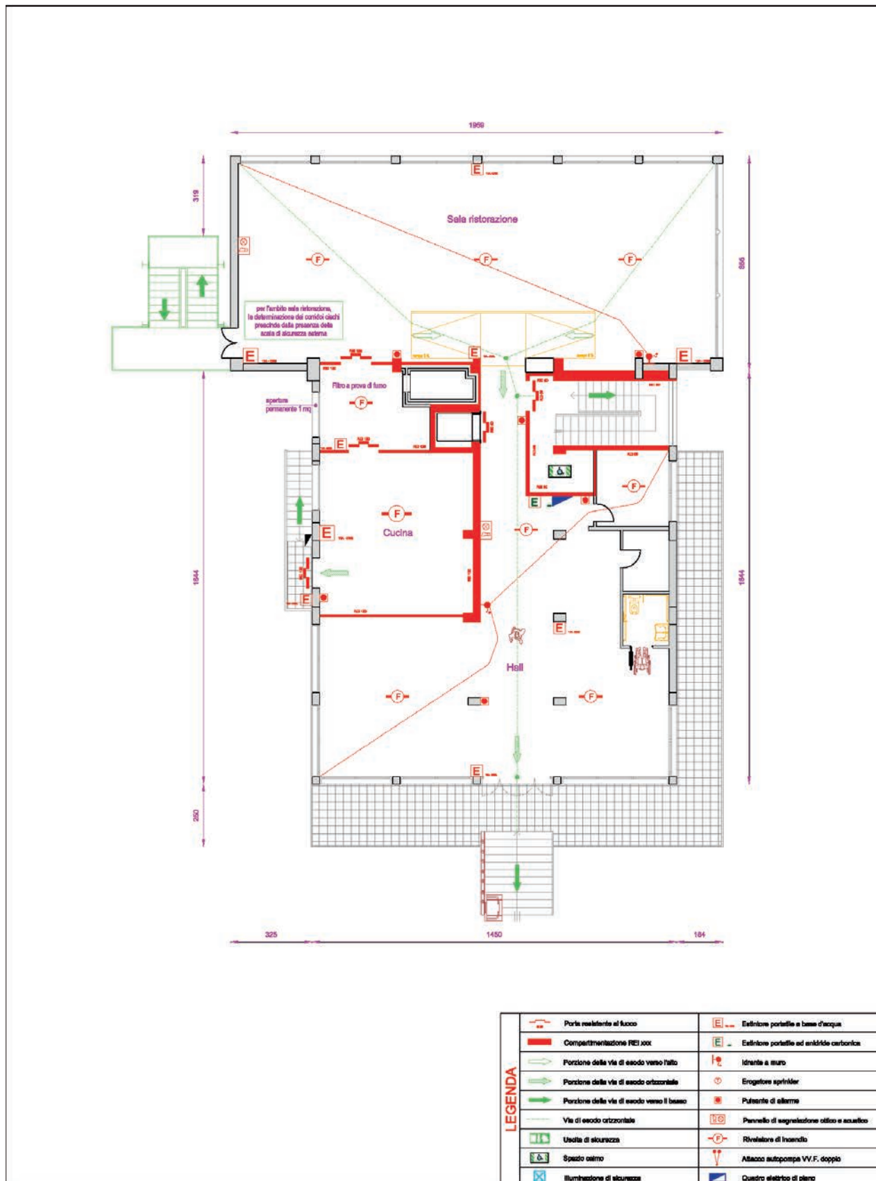
PLANIMETRIA - POST OPERAM - DEL PIANO PRIMO
